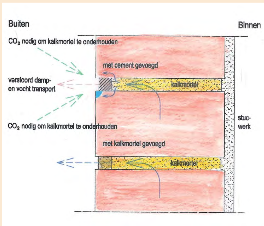
Een schematische tekening toont de problemen, die bij het gebruik van verkeerde mortels ontstaan.
